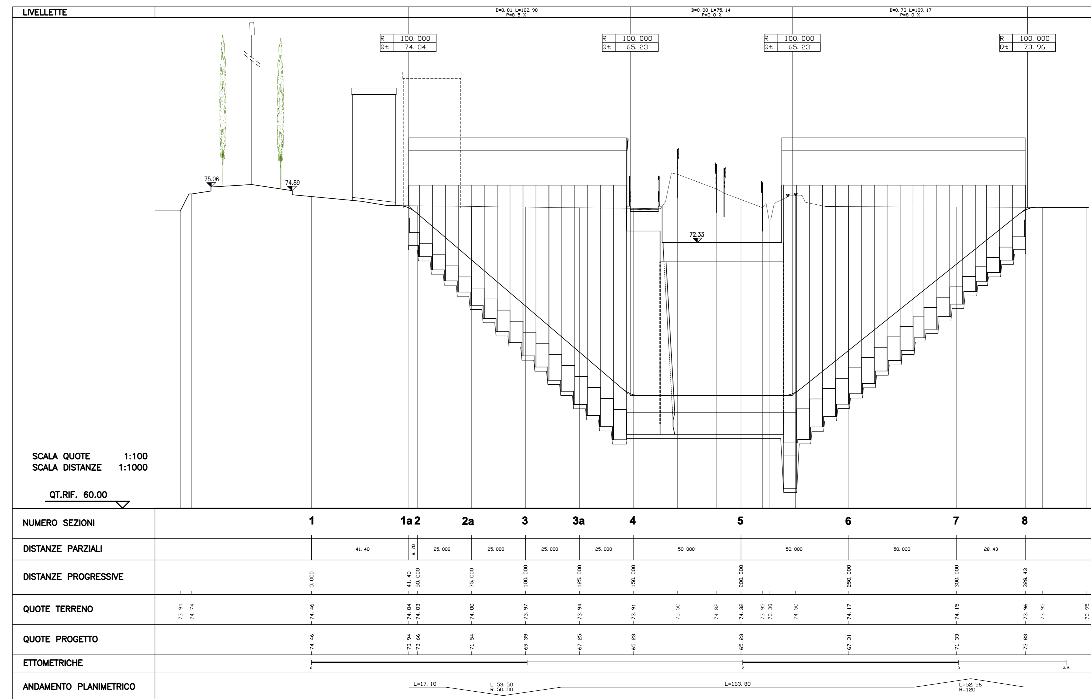
PROFILO LONGITUDINALE SOLUZIONE 3 SCALA 1:1000/100
