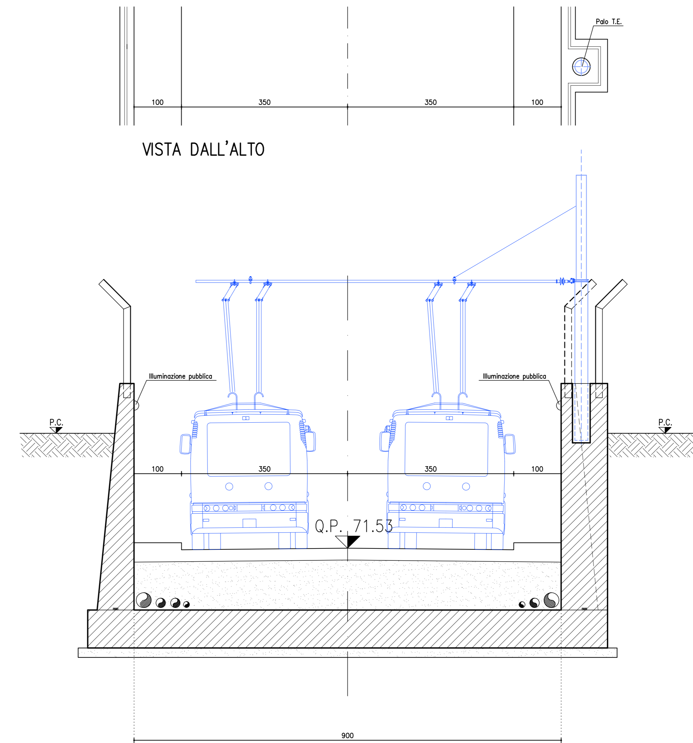
SEZIONE TRASVERSALE MURO AD "U" (2a-2a) IN CORRISPONDENZA PREDISPOSIZIONE PALO T.E. SCALA 1:50
