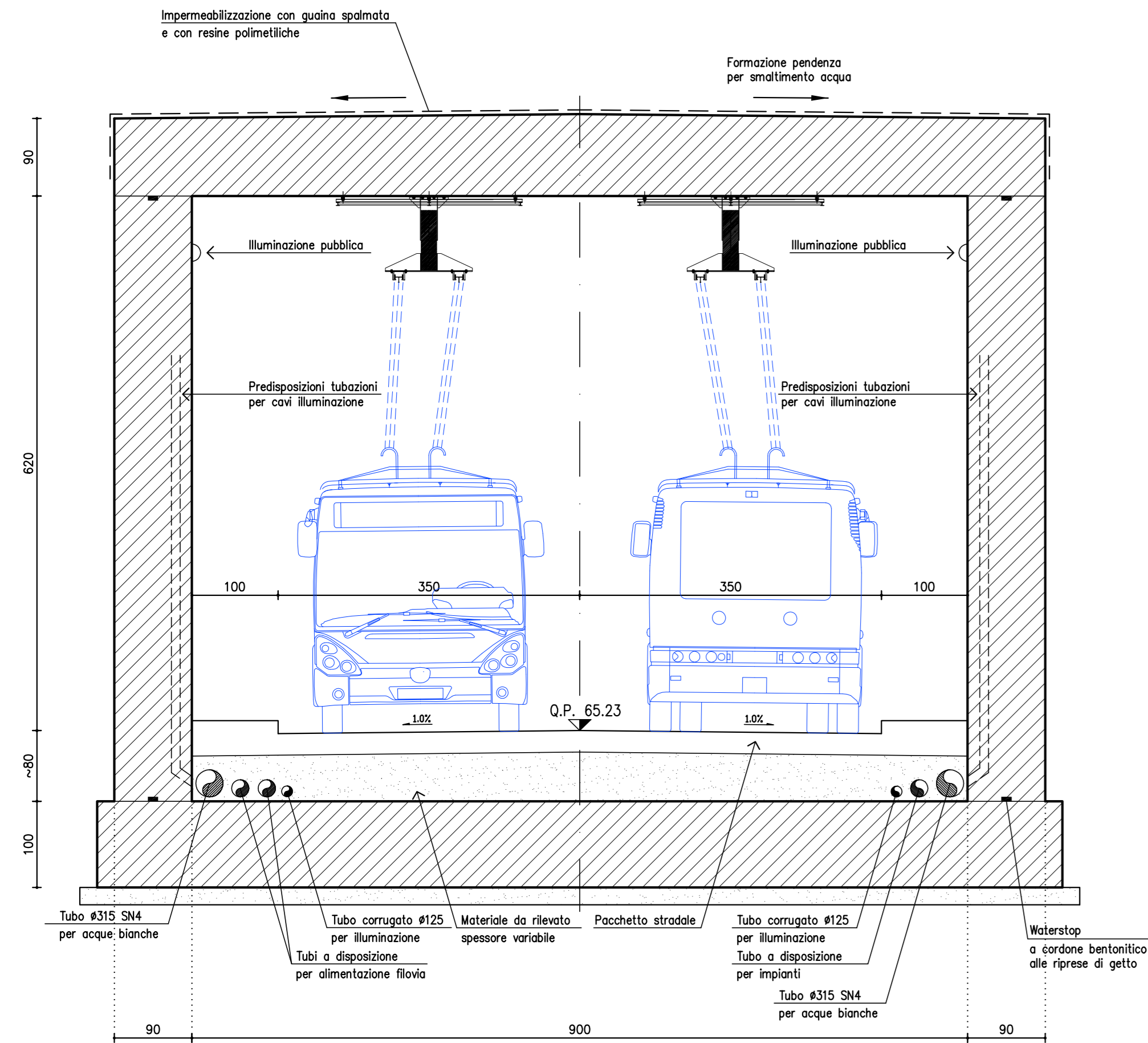
SEZIONE TRASVERSALE MANUFATTO SOTTOTANGENZIALE SCALA 1:50
