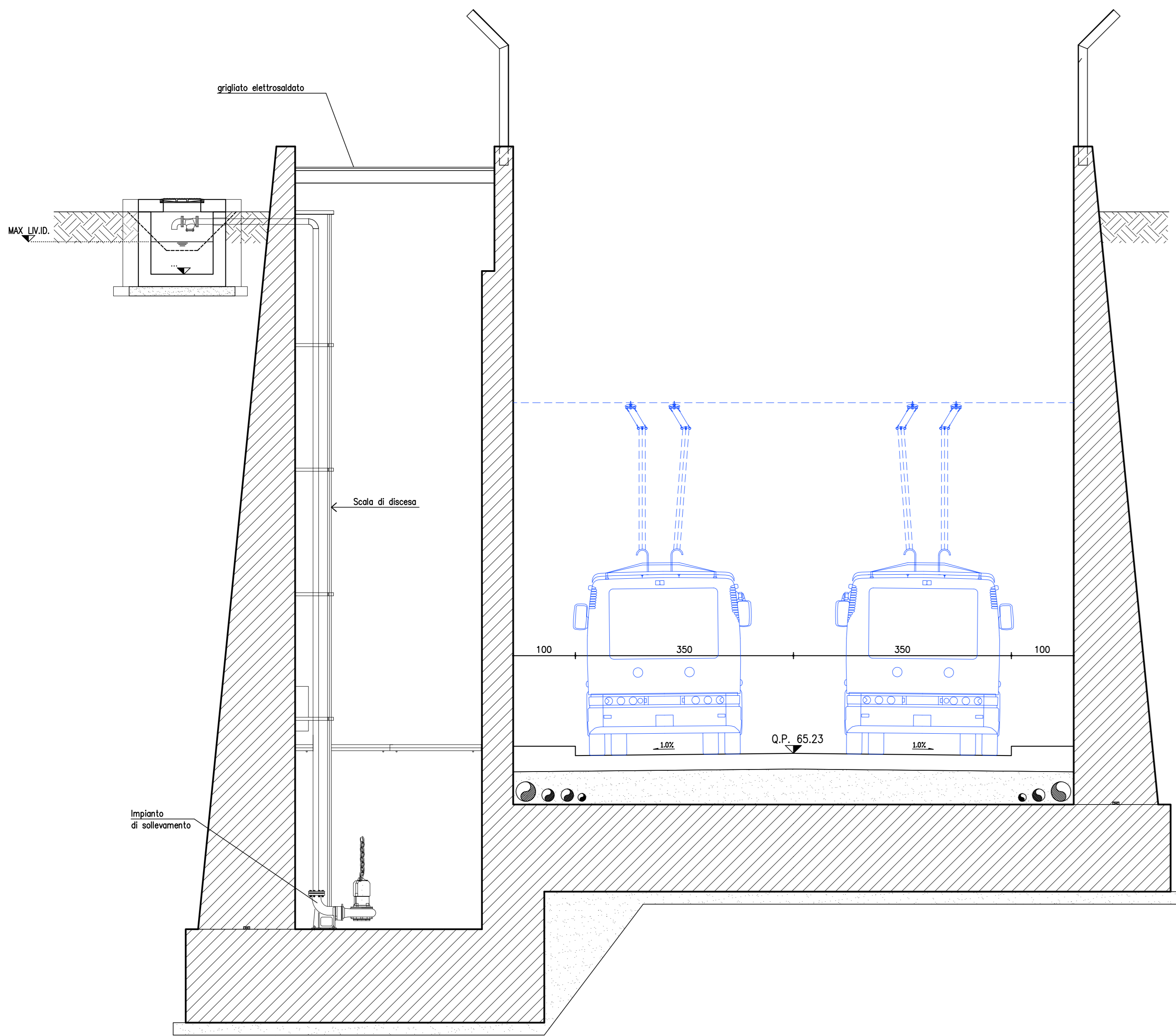
SEZIONE IN CORRISPONDENZA VASCA DI SOLLEVAMENTO SCALA 1:50
