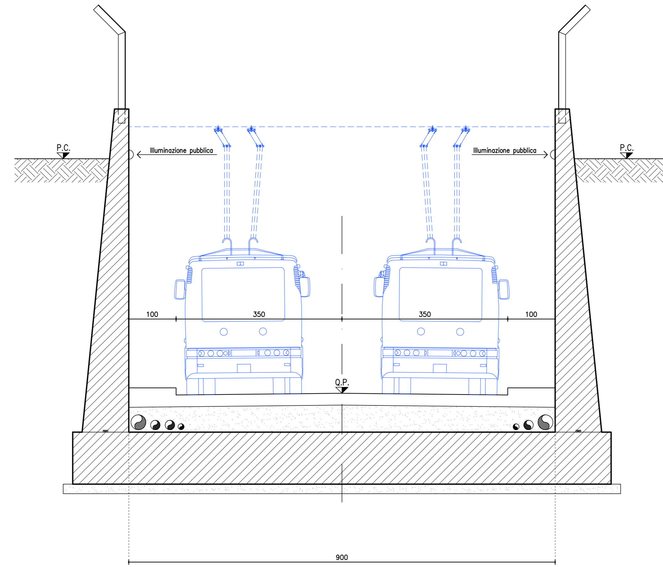
SEZIONE TRASVERSALE TIPO MURO AD "U" SCALA 1:50
